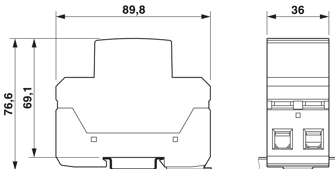
Rysunek wymiarowy
