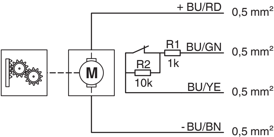
Rysunek schematyczny
