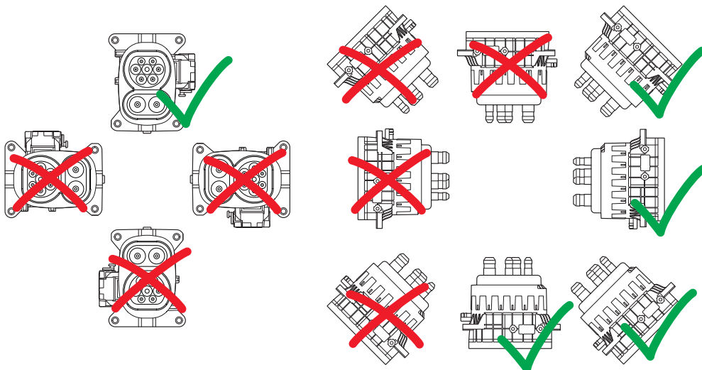
rysunek złączy
