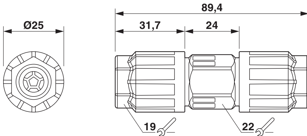
Rysunek wymiarowy
