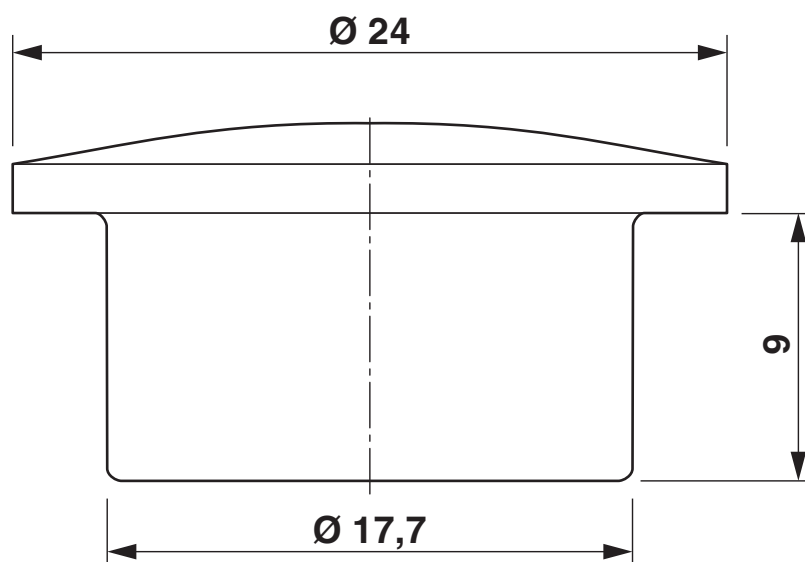
Rysunek wymiarowy
