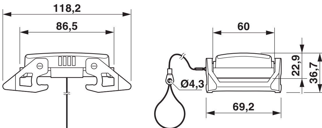
Rysunek wymiarowy
