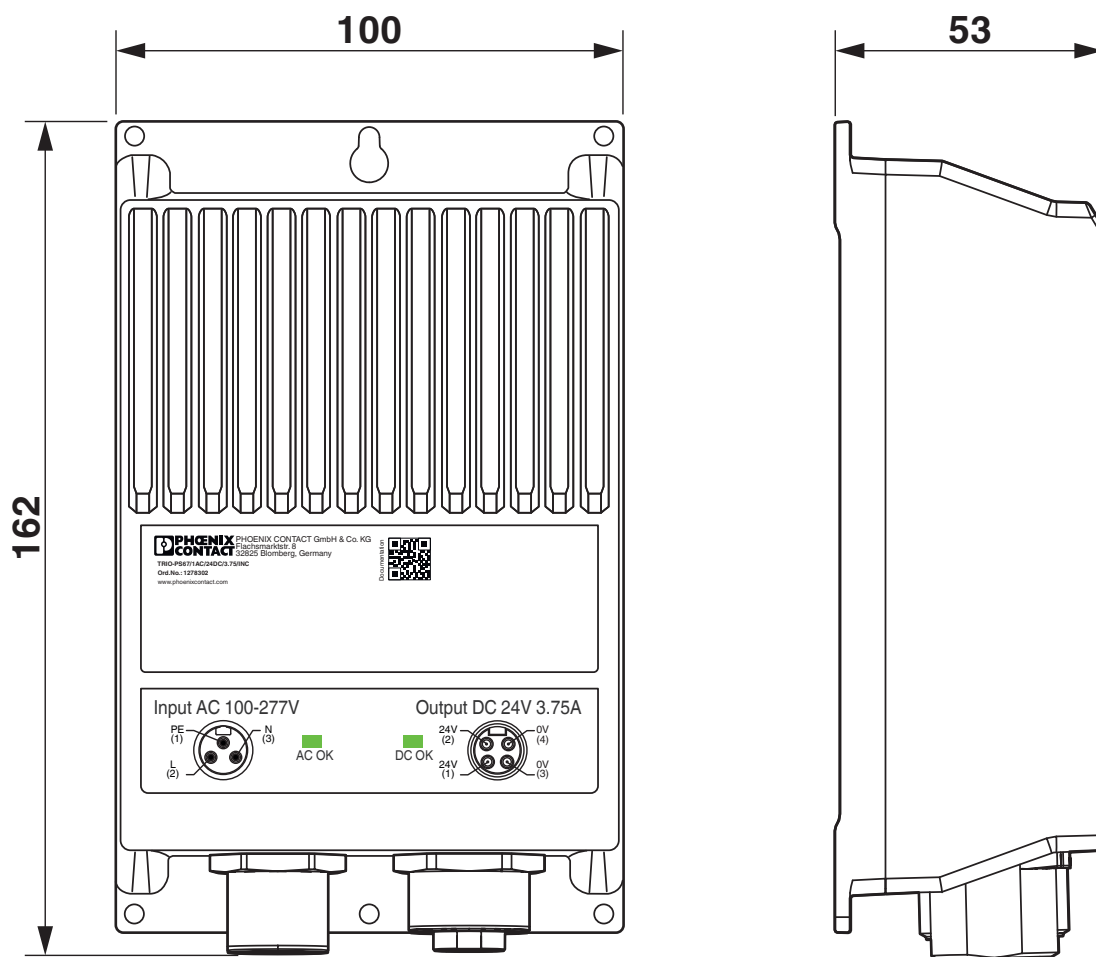
Rysunek wymiarowy
