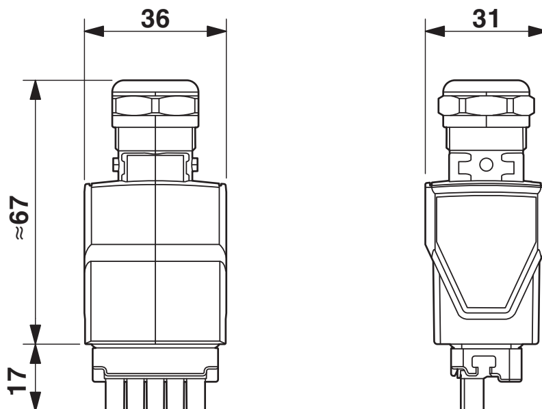
Rysunek wymiarowy
