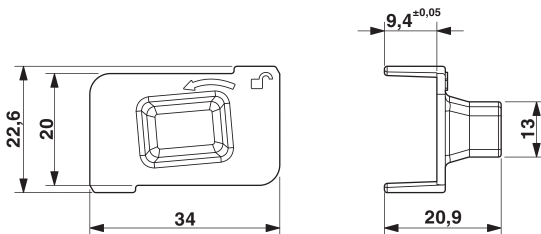
Rysunek wymiarowy
