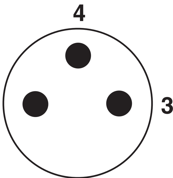
Układ styków, wtyk M8, 3-biegunowy, widok od strony styków
