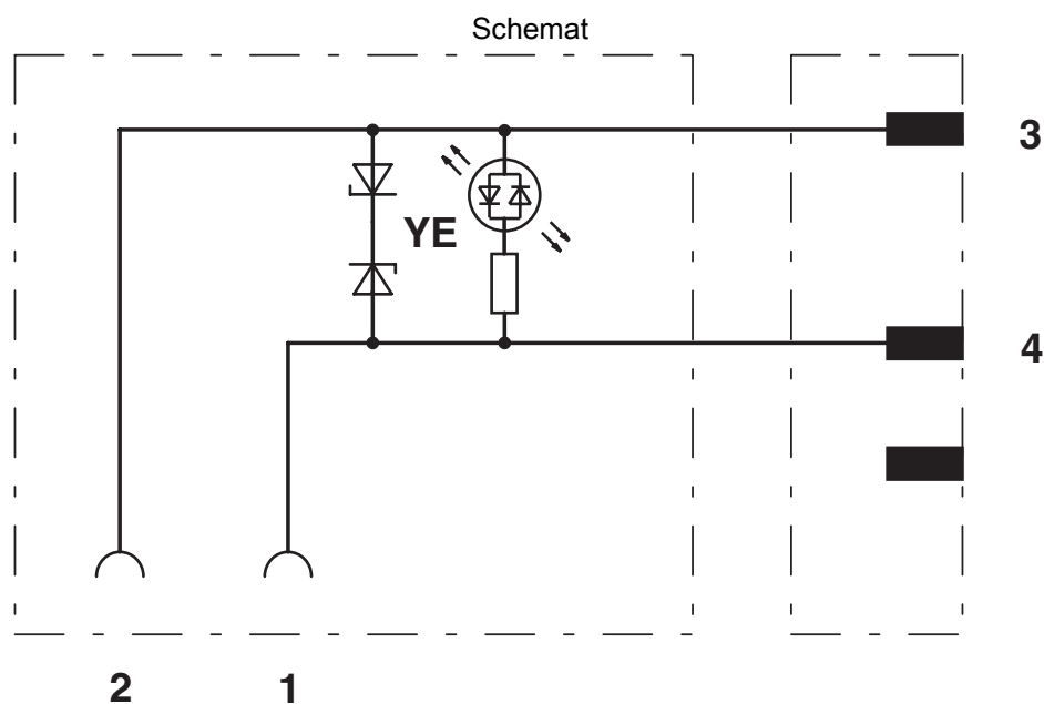
Rysunek schematyczny
