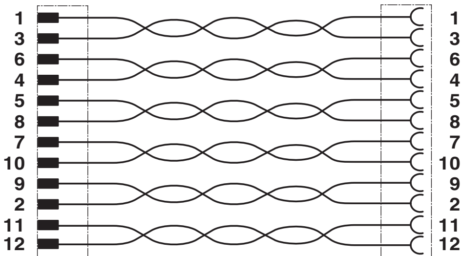
Schemat
