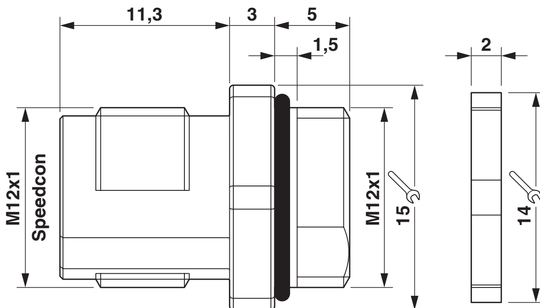
Rysunek wymiarowy
