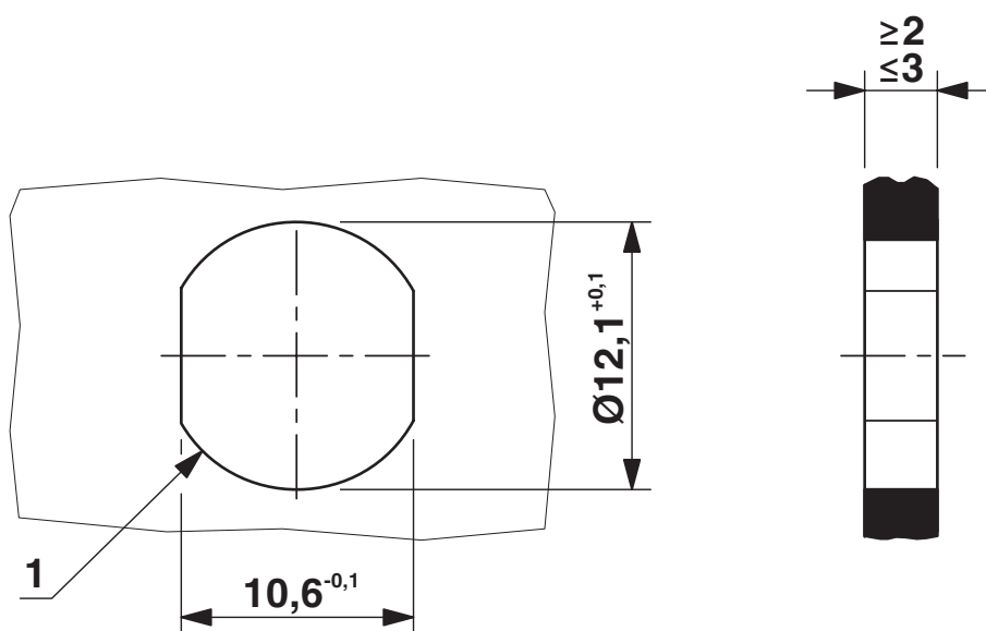
Rysunek wymiarowy
