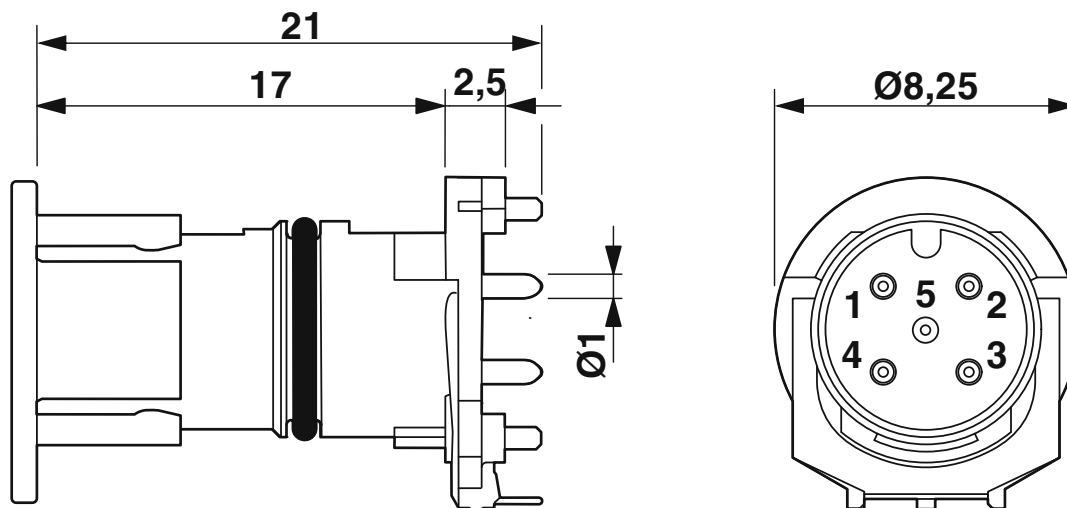
Rysunek wymiarowy
