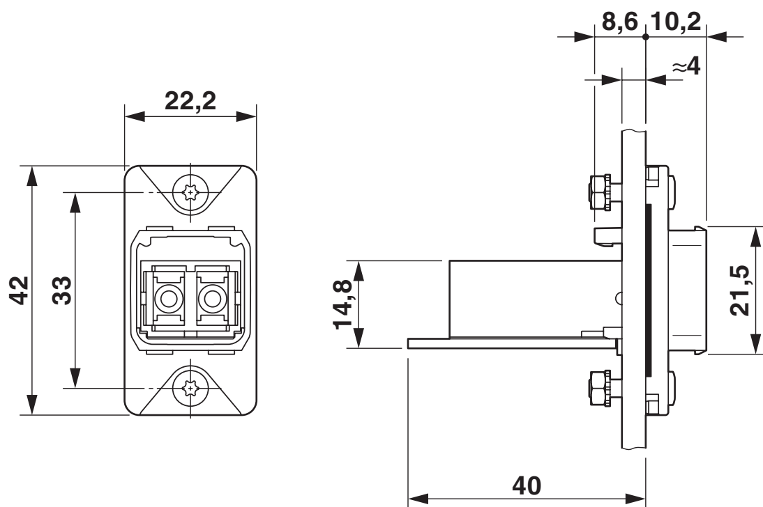
Rysunek wymiarowy
