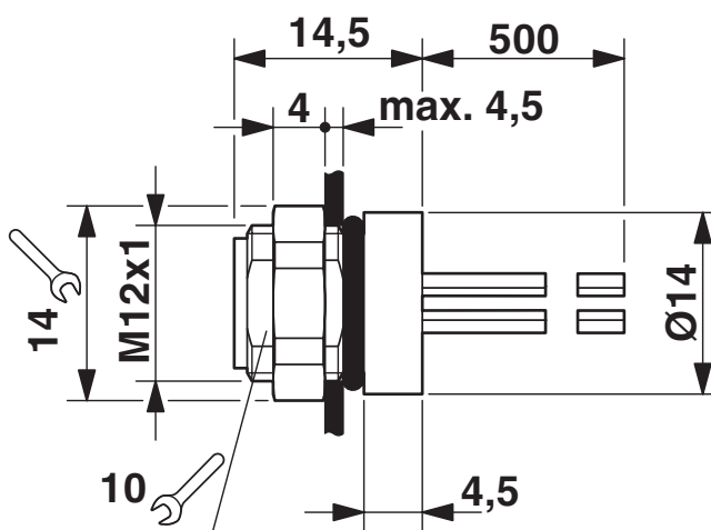
Rysunek wymiarowy
