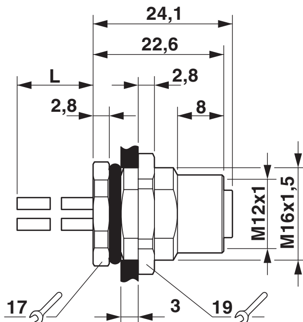
Rysunek wymiarowy
