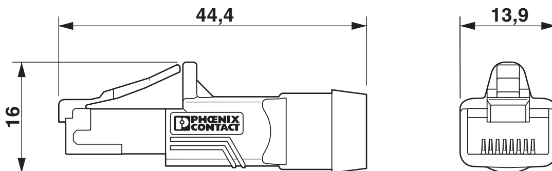
Rysunek wymiarowy
