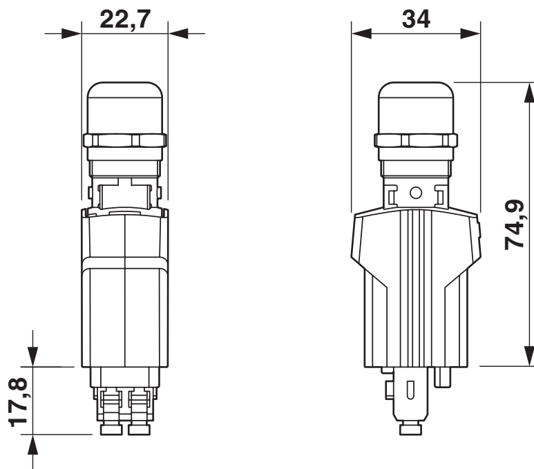
Rysunek wymiarowy
