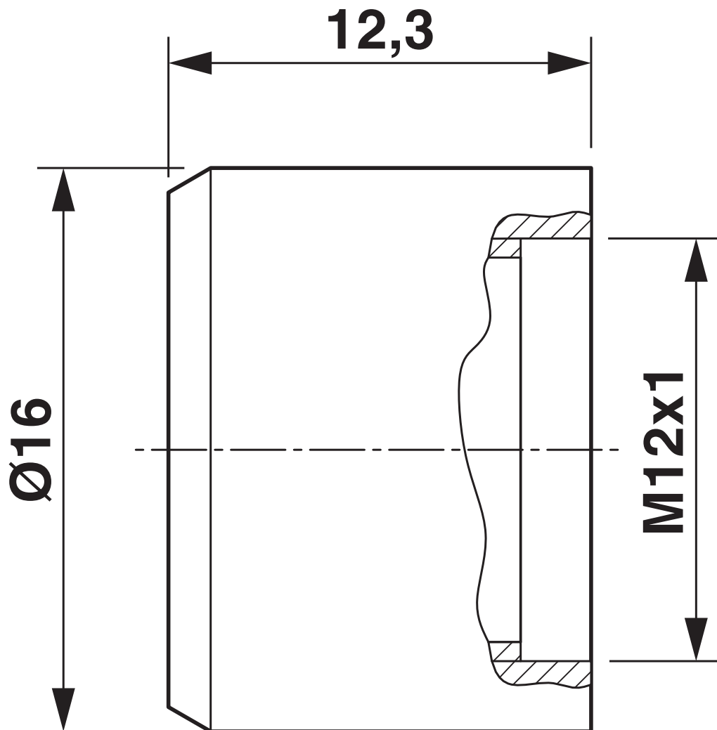
Rysunek wymiarowy
