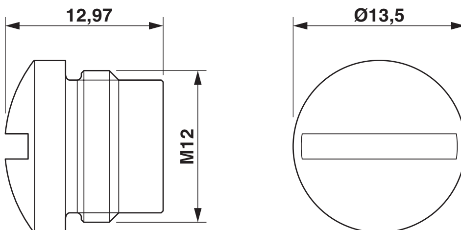
Rysunek wymiarowy
