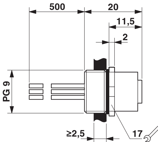
Rysunek wymiarowy
