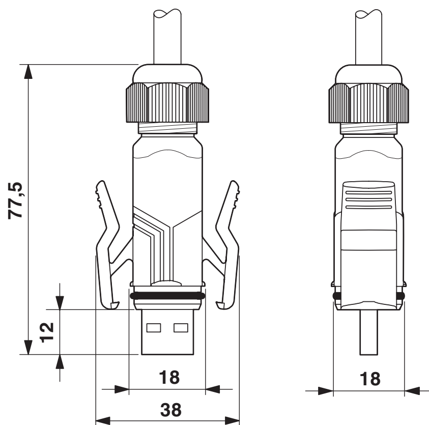
Rysunek wymiarowy
