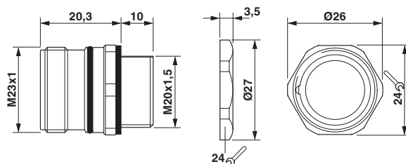
Rysunek wymiarowy
