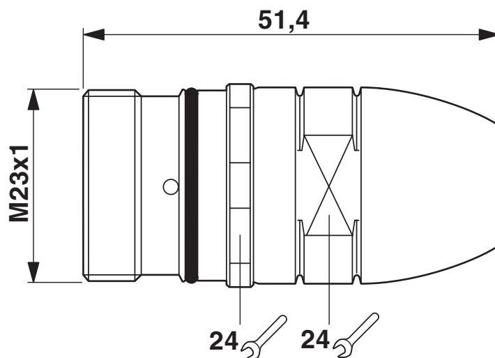
Rysunek wymiarowy
