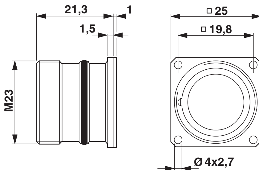
Rysunek wymiarowy
