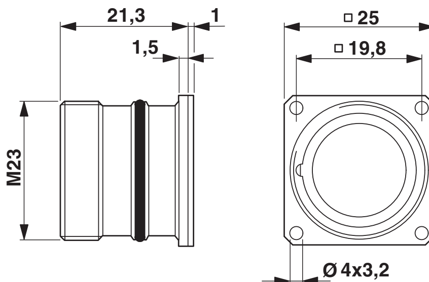
Rysunek wymiarowy
