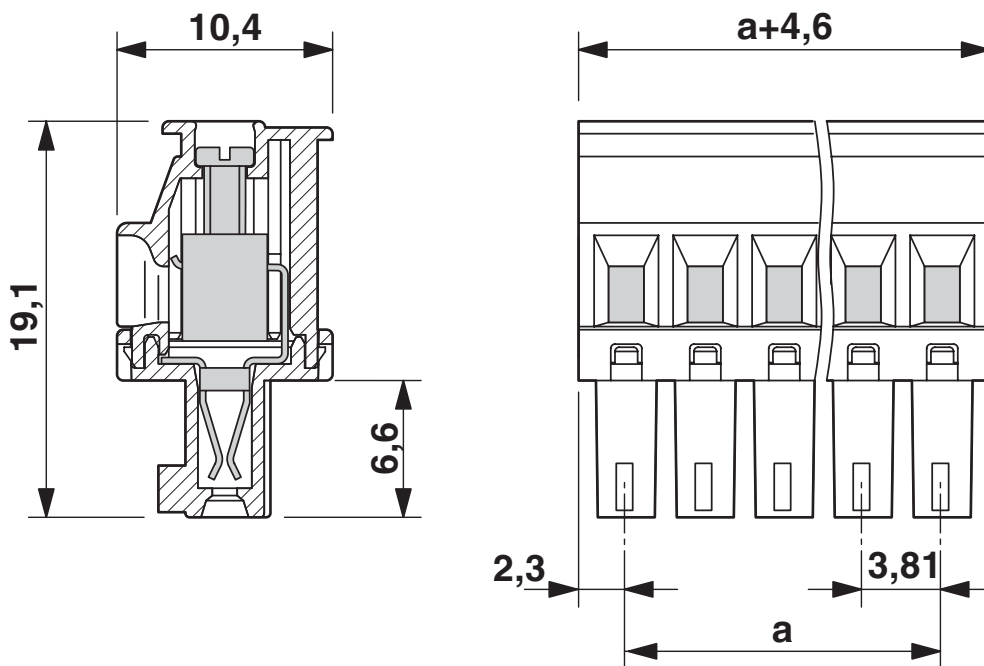
Rysunek wymiarowy
