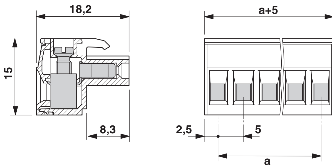
Rysunek wymiarowy
