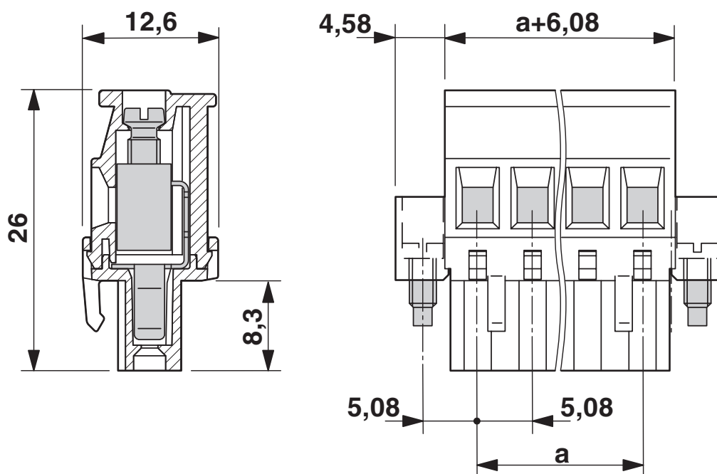
Rysunek wymiarowy
