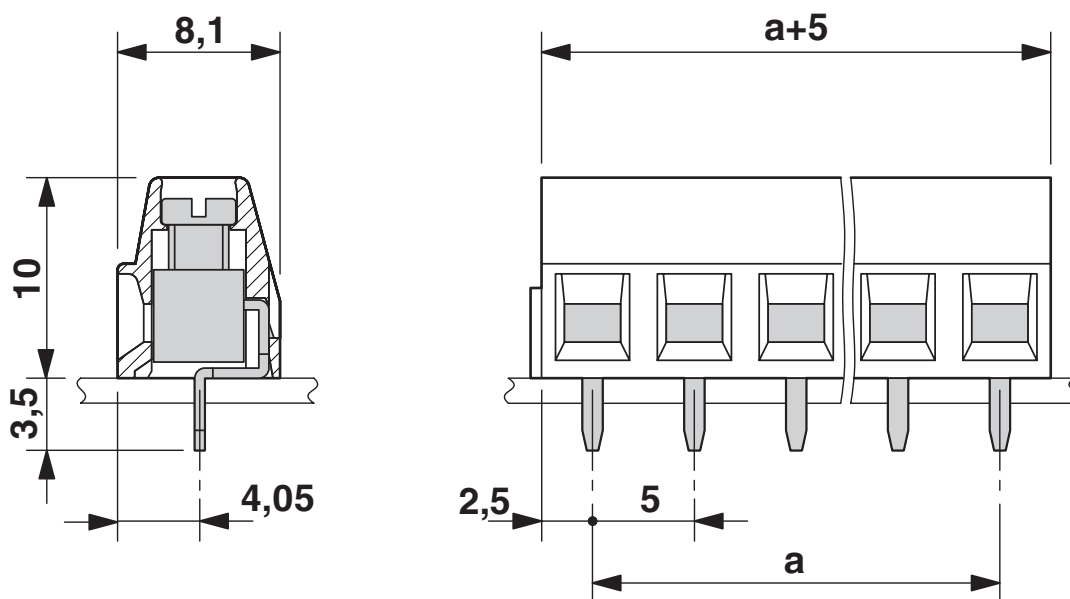
Rysunek wymiarowy
