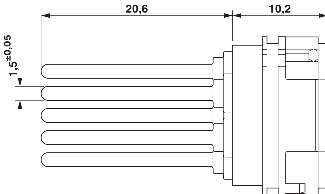
Rysunek wymiarowy
