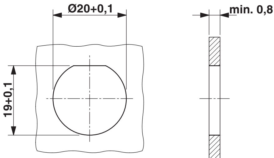
Rysunek wymiarowy
