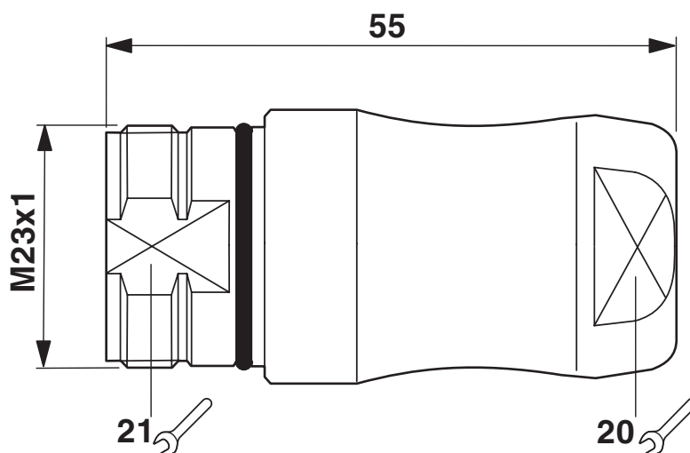
Rysunek wymiarowy
