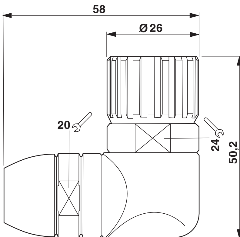
Rysunek wymiarowy
