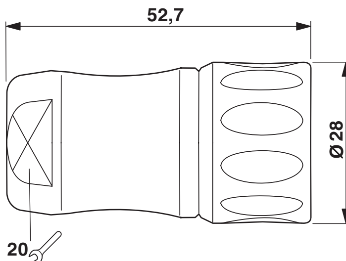
Rysunek wymiarowy
