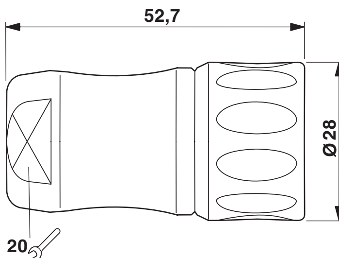
Rysunek wymiarowy
