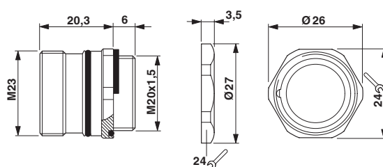
Rysunek wymiarowy
