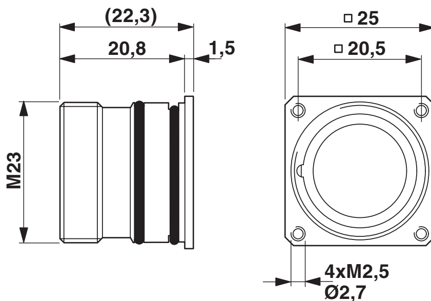
Rysunek wymiarowy
