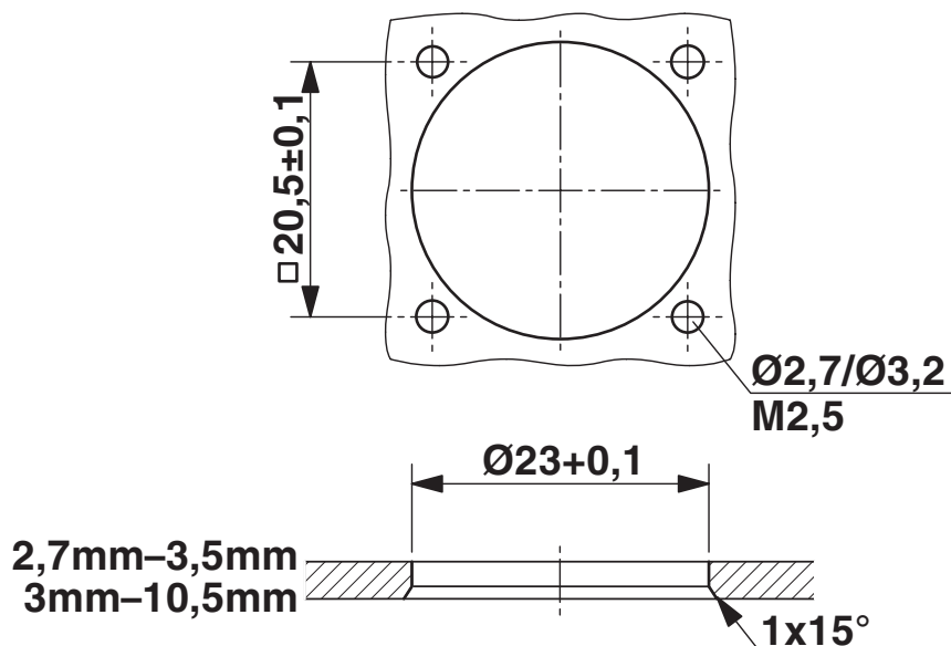
Rysunek wymiarowy
