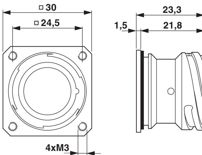
Rysunek wymiarowy
