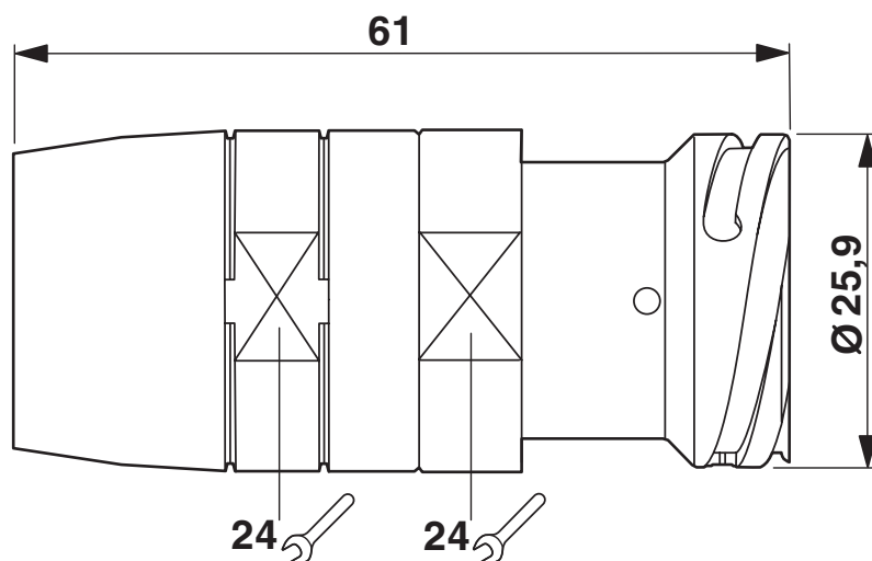
Rysunek wymiarowy
