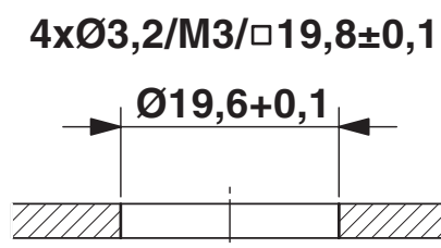
Rysunek wymiarowy
