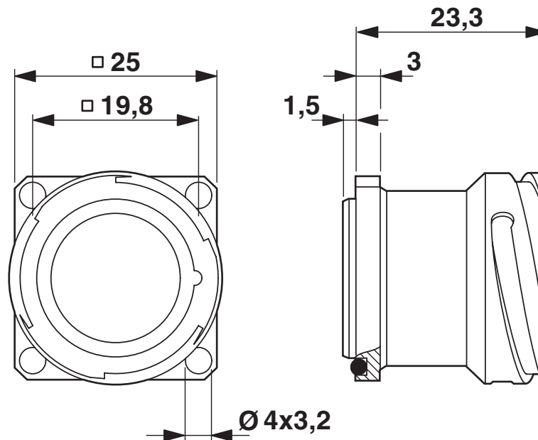
Rysunek wymiarowy
