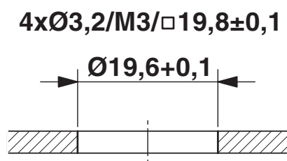
Rysunek wymiarowy
