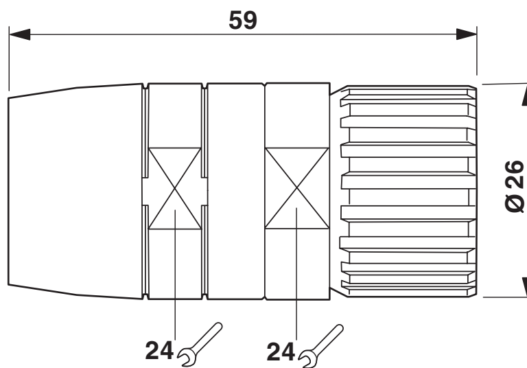
Rysunek wymiarowy
