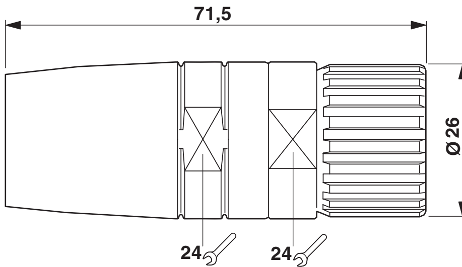
Rysunek wymiarowy
