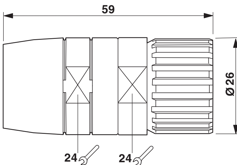
Rysunek wymiarowy
