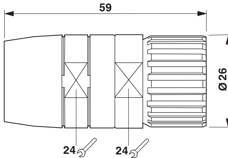
Rysunek wymiarowy
