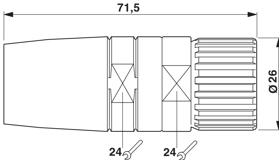
Rysunek wymiarowy
