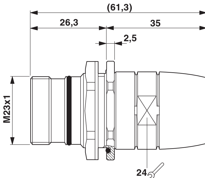
Rysunek wymiarowy
