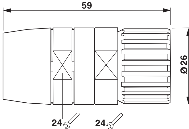
Rysunek wymiarowy
