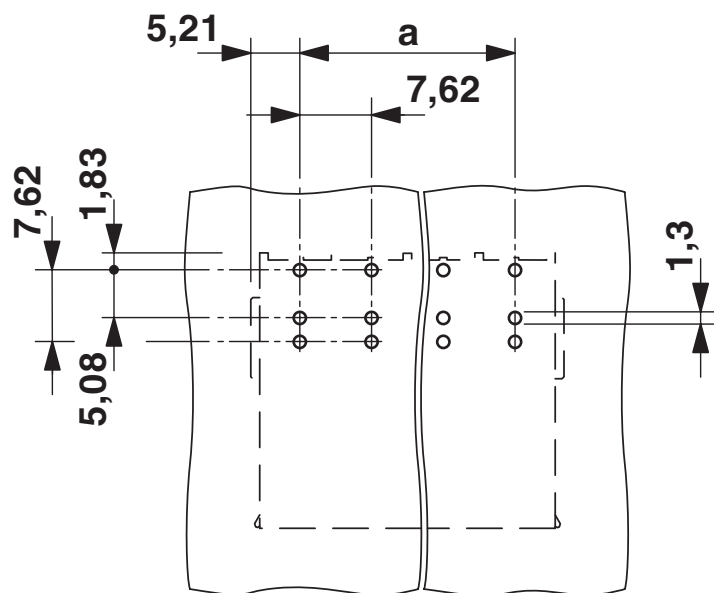
Otworowanie/geometria płytek lutowicznych
