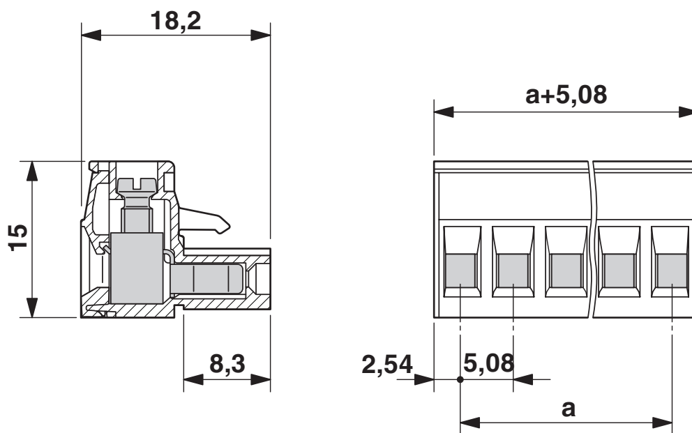
Rysunek wymiarowy
